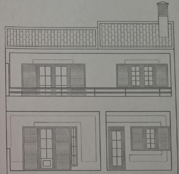
ALÇADO POSTERIOR
