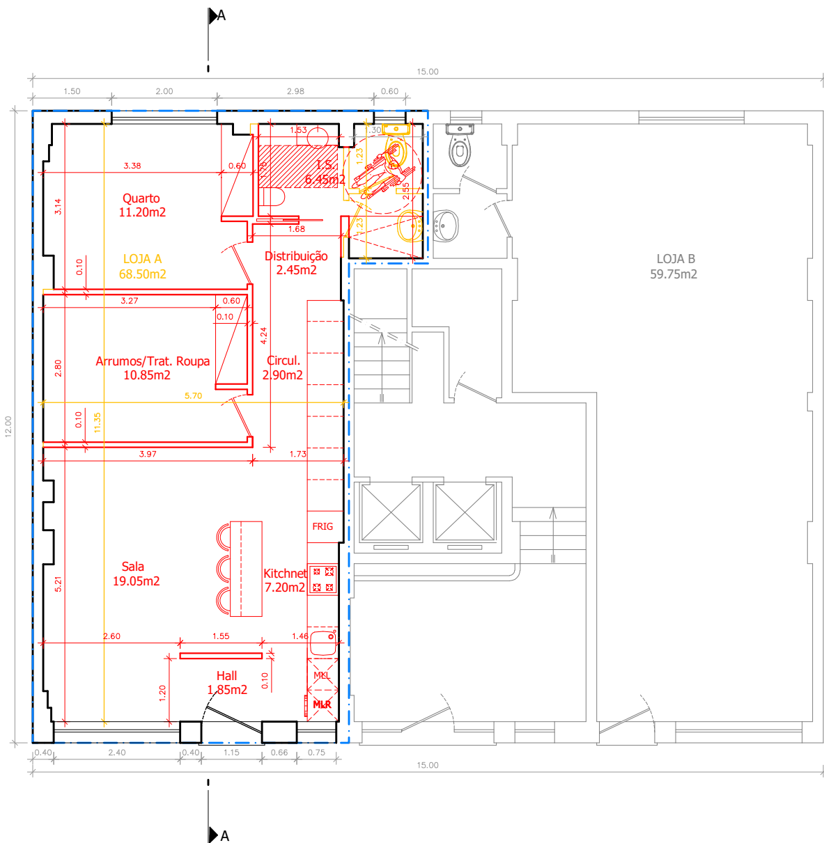
PLANTA DA FRAÇÃO
