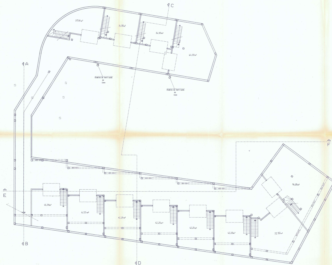
PLANTA DA CAVE (garagens)
