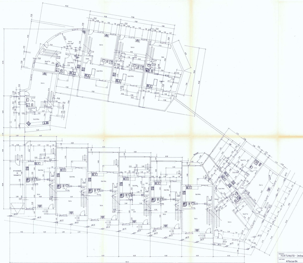
PLANTA DO RES-DO-CHÃO
