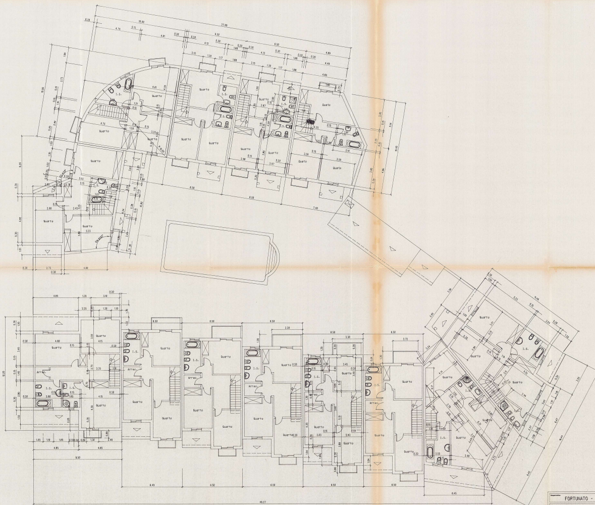
PLANTA 1º ANDAR
