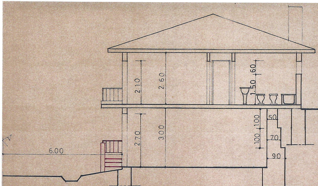
CORTE A-B
